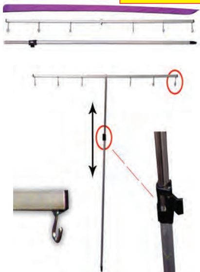
ART. 533240 PICCHETTO PORTACALAMENTI CON OCCHIELLO telescopico in alluminio, leggero e robusto. Altezza: aperto cm. 160, chiuso cm. 85. Telescopic aluminum rod holder for PORTACALAMENTI, it is light and strong. Length: opened 160 cm, closed 85 cm.
