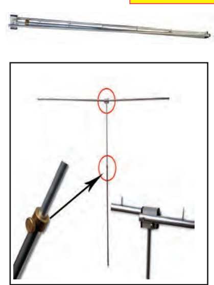
ART. 533250 PICCHETTO PORTACALAMENTI A SPILLO telescopico in alluminio, leggero e robusto. Altezza: aperto cm. 160, chiuso cm. 85. Telescopic aluminum rod holder for PORTACALAMENTI, it is light and strong. Length: opened 160 cm, closed 85 cm.
